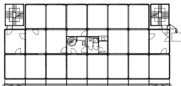
NIVEAU +2
