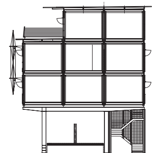
COUPE
